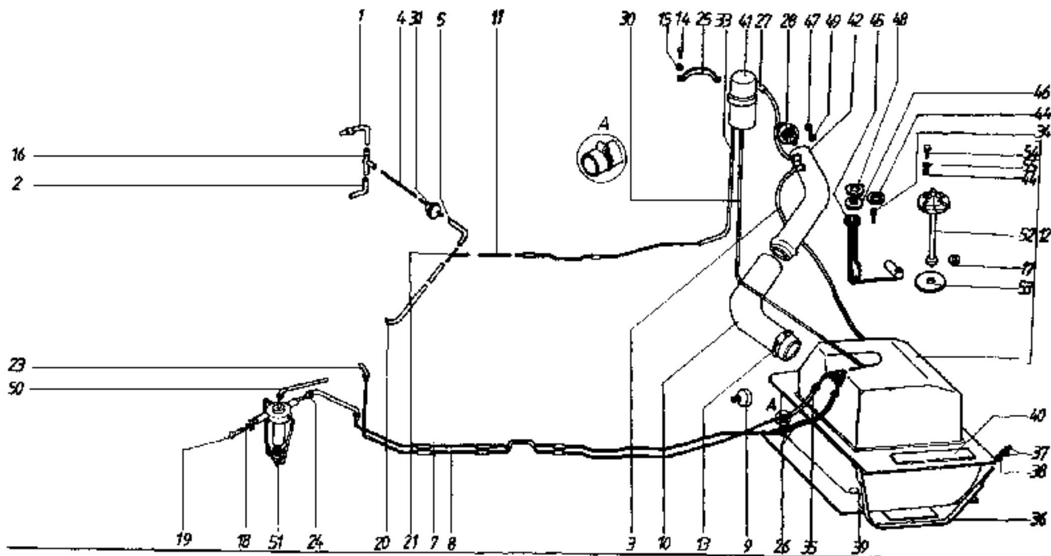
INSTALAȚIA DE ALIMENTARE
