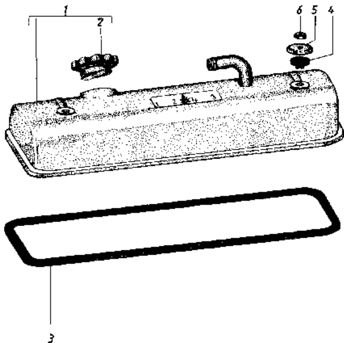
Couvercle Culasse L 25
